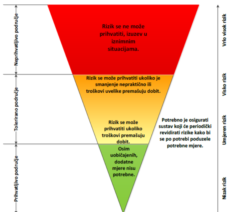
Slika 27: – ALARP načela
